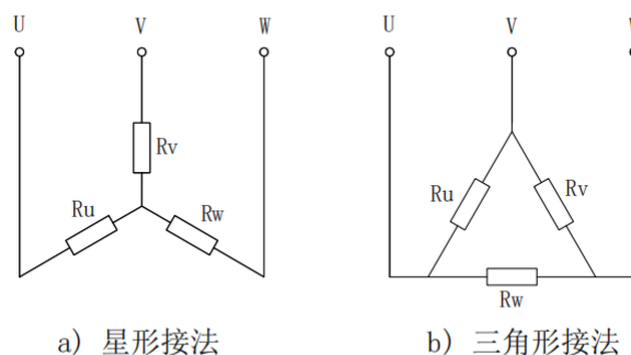
图2 三相绕组接线示意图
