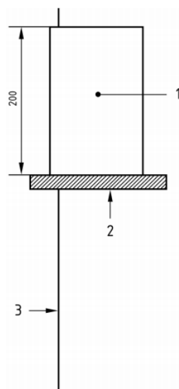
1—完整电缆；2—固定装置；3—承拉元件
