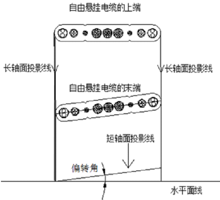
图A. 2 自由悬挂偏转角测量示意图
