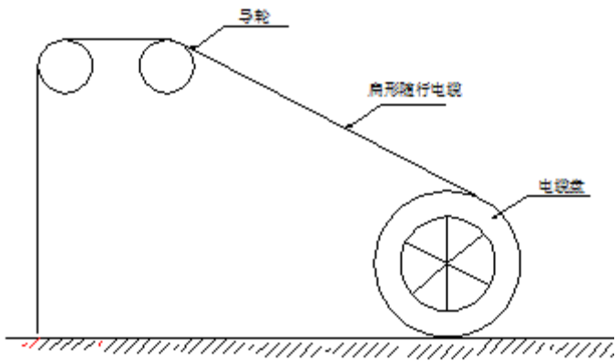
图A. 1 自由悬挂偏转角示意图
