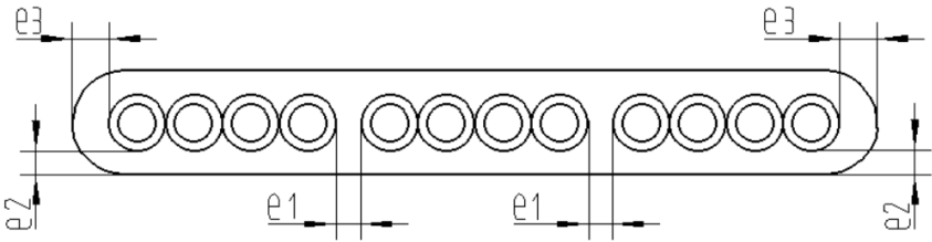
图1 组间间距和护套厚度截面图
