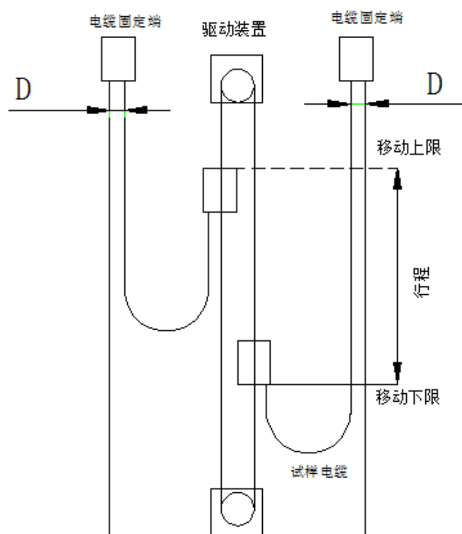
图B.1 运行时平稳性试验示意图
