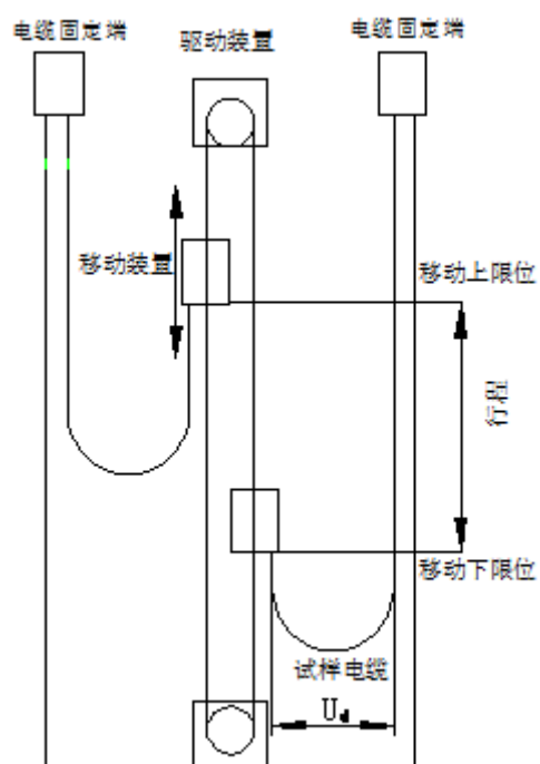
图C.1 成品疲劳运行模拟试验装置示意图
