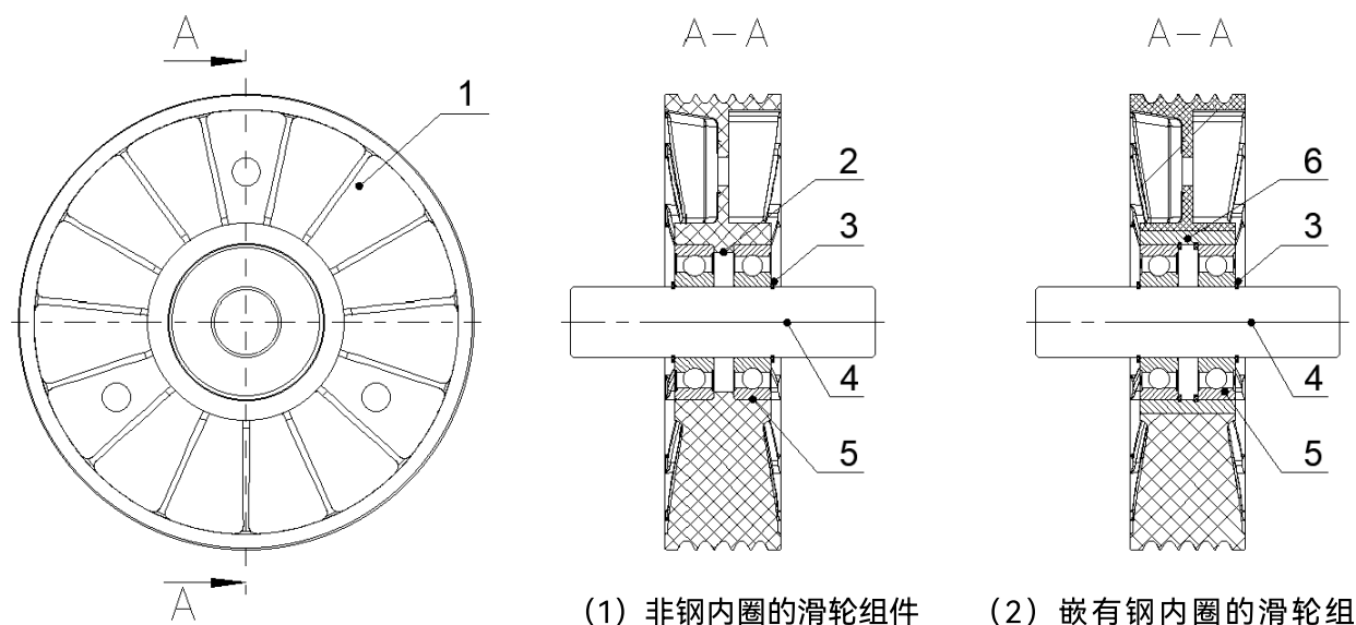
图 1 滑轮组件示意图
