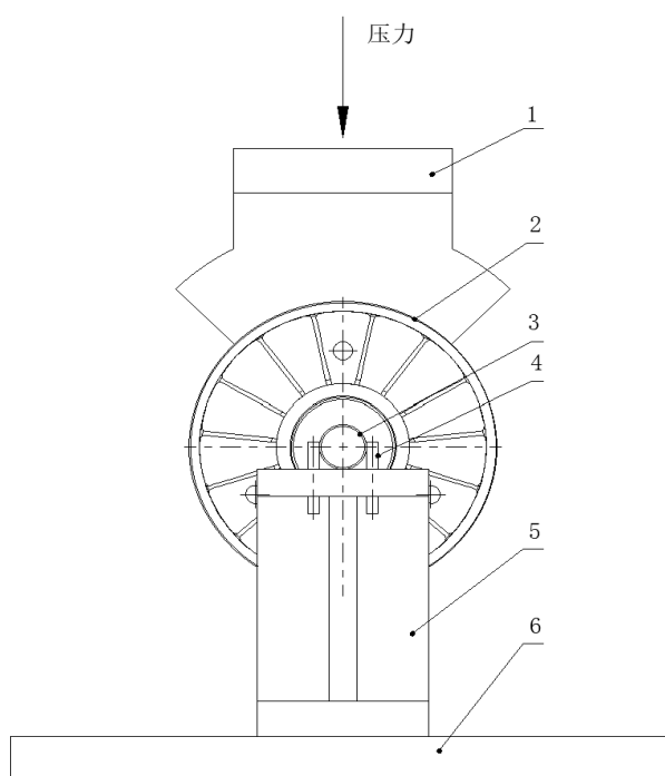
图 4 压力试验机示意图
