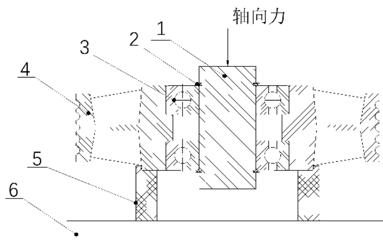
图 6 轴向力测试试验机示意图（非钢内圈滑轮组件）
