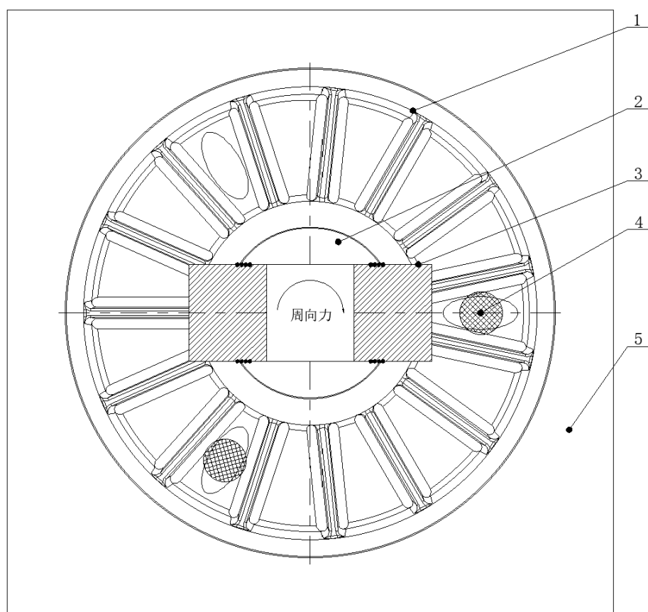
图 8 周向扭矩试验示意图
