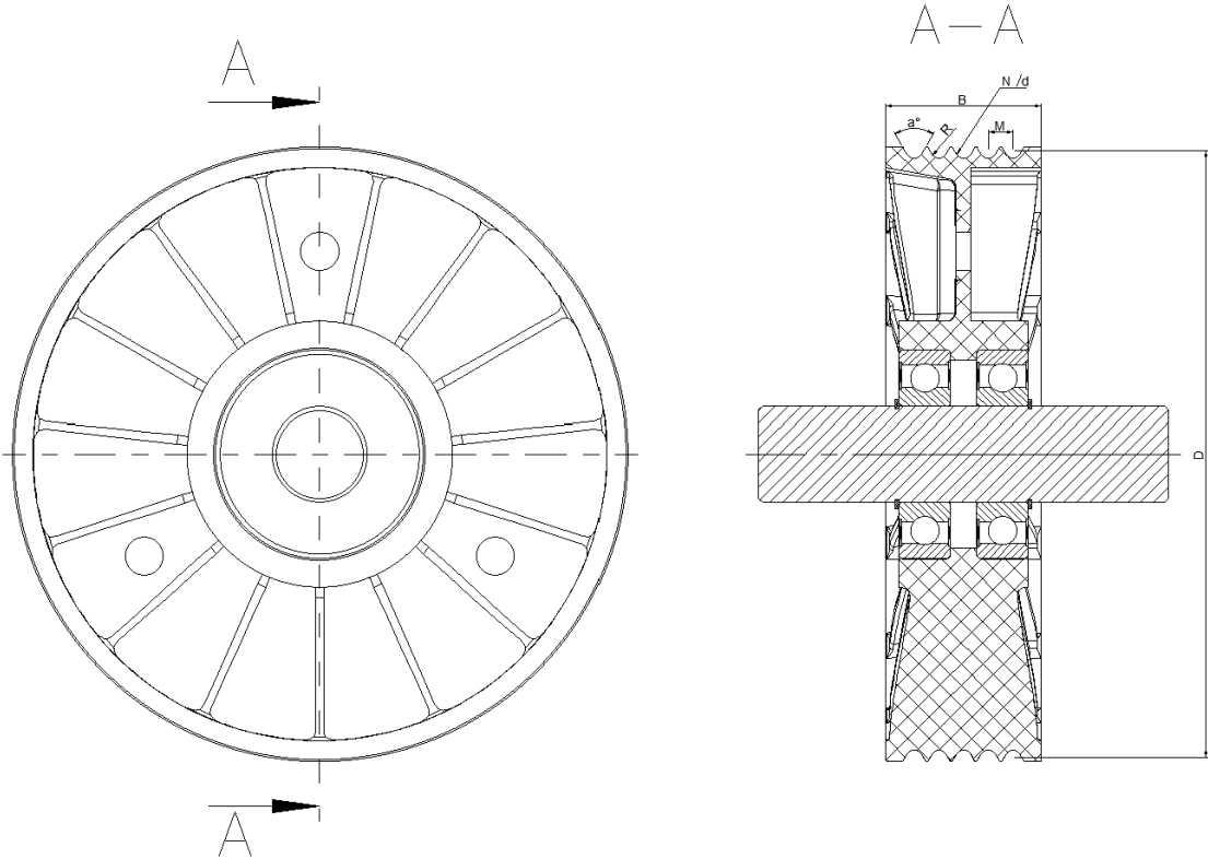
图 B.1 典型滑轮示意图
