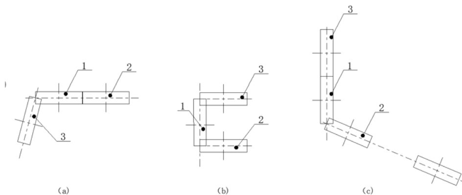
图 A.2 典型的电梯滑轮布局示意简图
