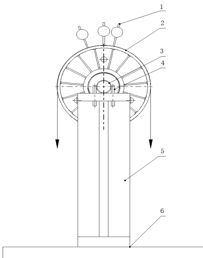
图 5 拉力试验机示意图
