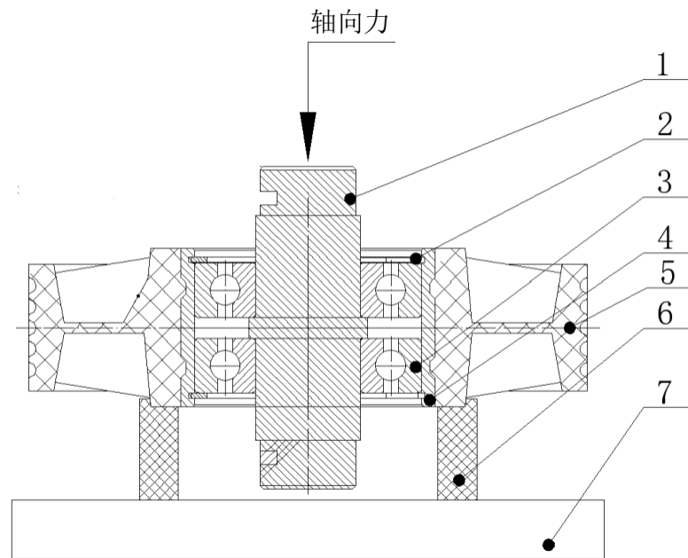
图 7 轴向力测试试验机示意图（嵌有钢内圈滑轮组件）
