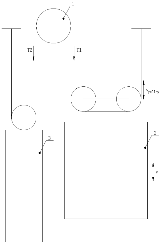
图 A.1 电梯系统示意图
