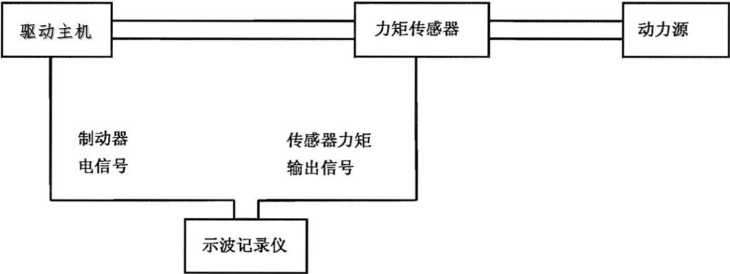
图 1 制动器制动响应时间检测示意图
