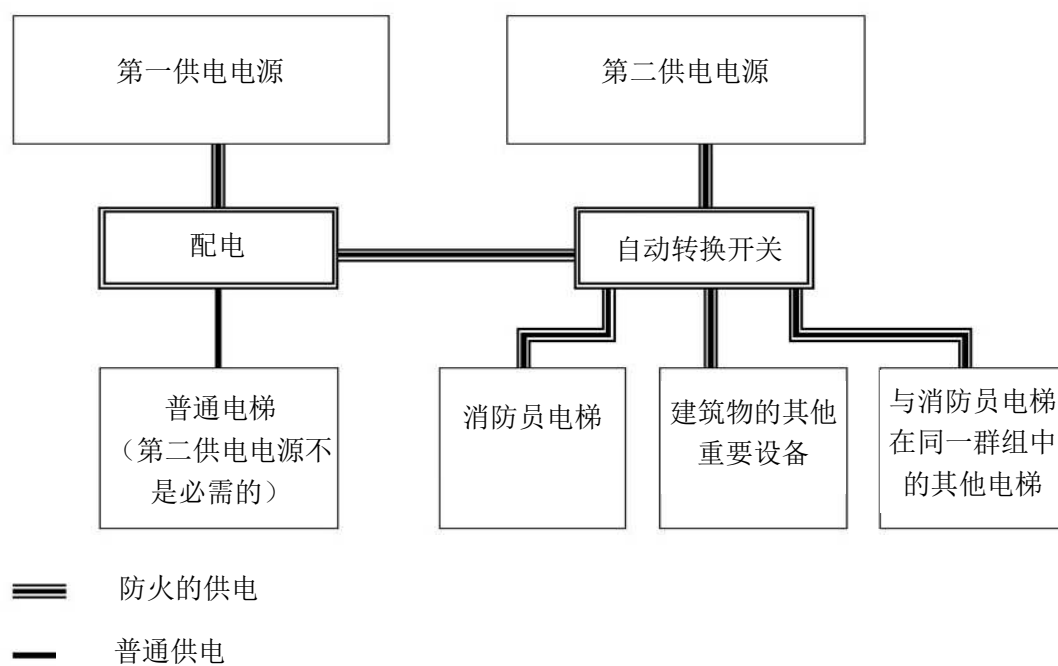
图 B.1 消防员电梯供电电源示例
