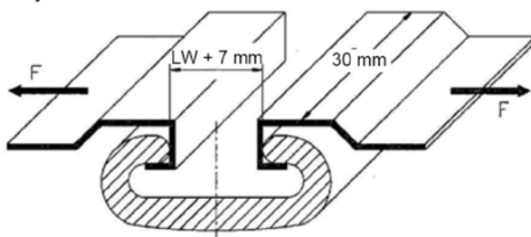
图5 扶手带唇口张力试验
