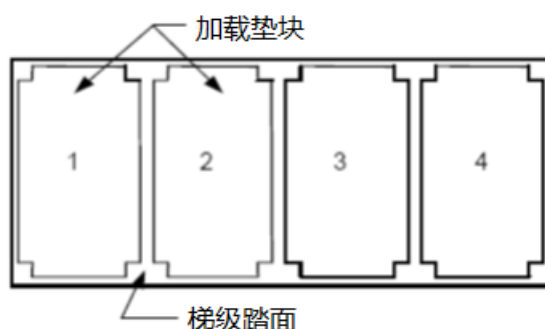
图 3 踏面静载分布载荷试验示意
