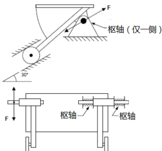
图 4 轴不同步位移试验
