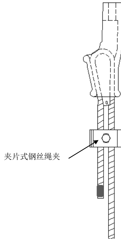
图 B.2 夹片式钢丝绳夹安装示例
