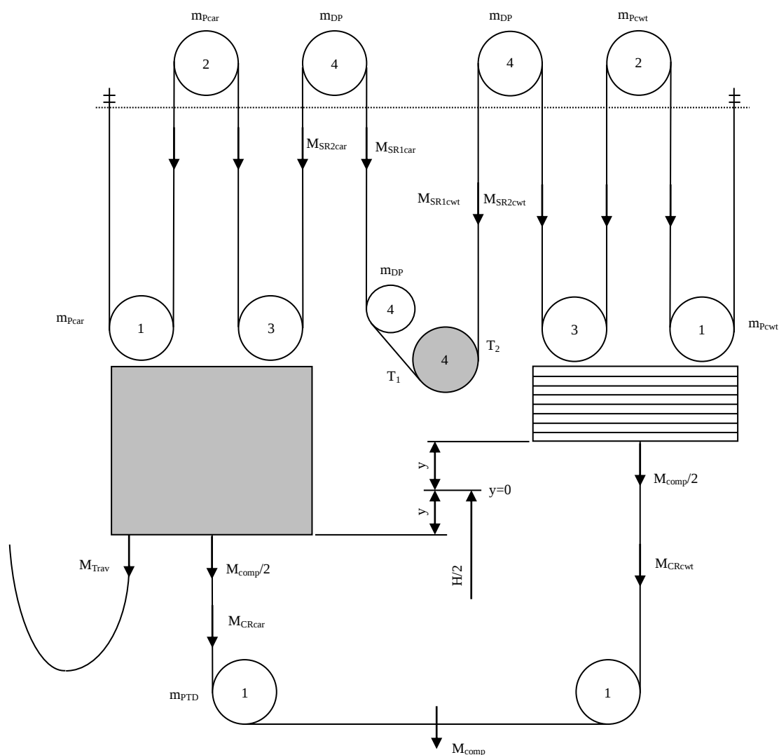
图 5 通常的曳引机下置情况
